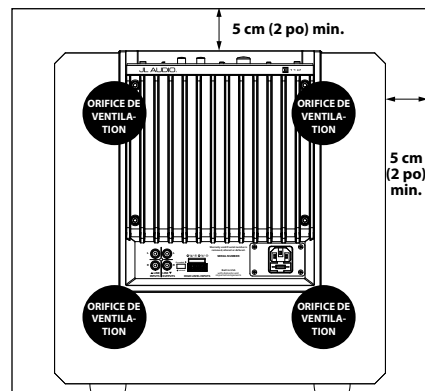
Vue arrière du boîtier :
