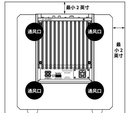
机柜安装背面视图:
