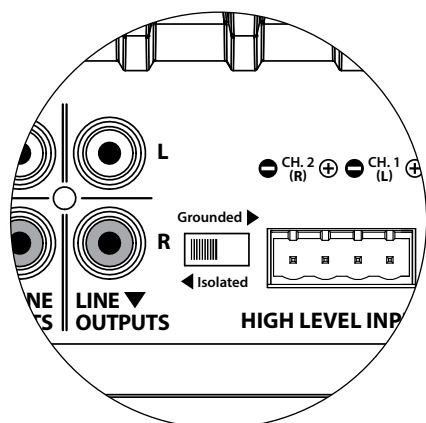
Gli ingressi a sinistra e a destra sull'E-Sub sono aggiunti internamente in un unico canale mono.
