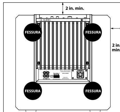
Visuale posteriore dell'installazione nella teca:
